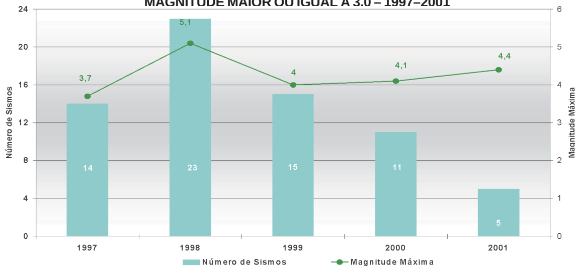
Gráfico 8.17 – EVOLUÇÃO DO NÚMERO ANUAL DE SISMOS BRASILEIROS COM MAGNITUDE MAIOR OU IGUAL A 3,0 – 1997–2001
