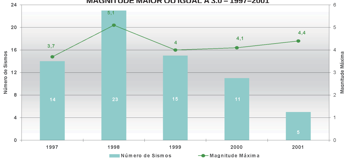
Gráfico 8.17 – EVOLUÇÃO DO NÚMERO ANUAL DE SISMOS BRASILEIROS COM MAGNITUDE MAIOR OU IGUAL A 3.0 – 1997–2001
