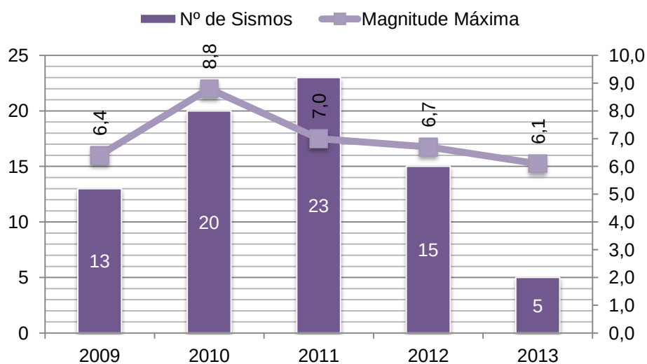
Gráfico 8.11 – Evolução do Número Anual de Sismos Brasileiros com Magnitude Maior ou Igual a 3,0, 2009 a 2013
