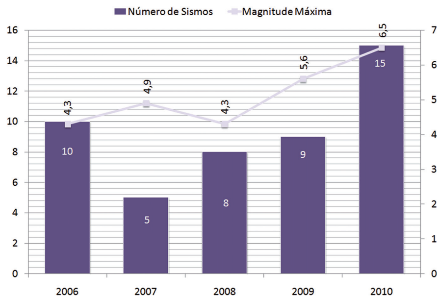
Gráfico 8.09: Evolução do Número Anual de Sismos Brasileiros com Magnitude Maior ou Igual a 3,0, 2006 a 2010
