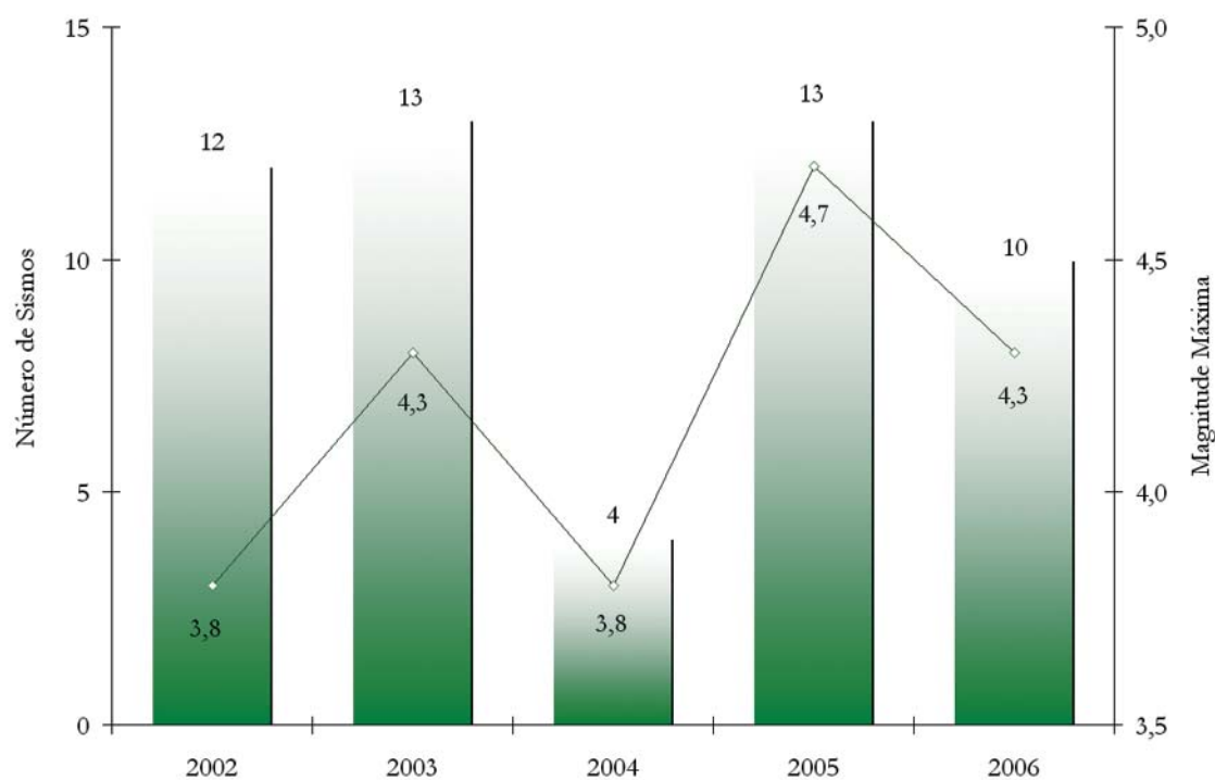
Gráfico 8.15: Evolução do Número Anual de Sismos Brasileiros com Magnitude Maior ou Igual a 3,0 – 2002–2006
